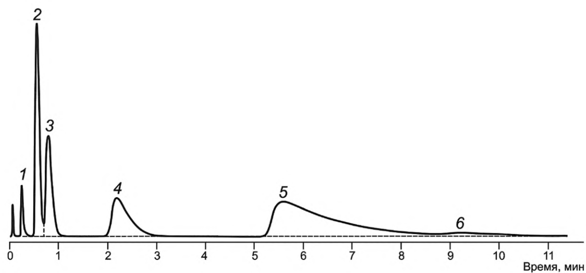
Рисунок Б.2 — Типовая хроматограмма растворителя марки 646
