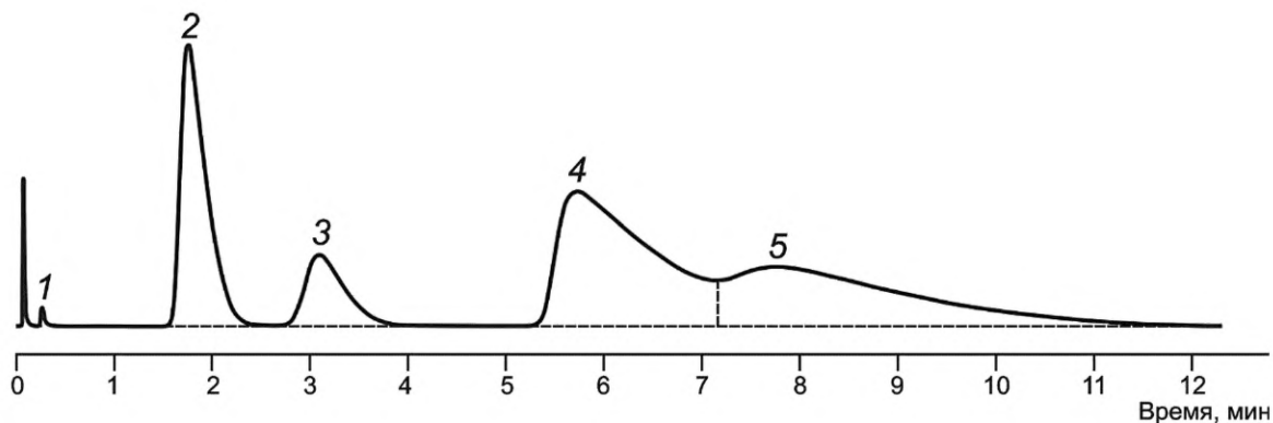
Рисунок Б.3 — Типовая хроматограмма растворителя марки 647
