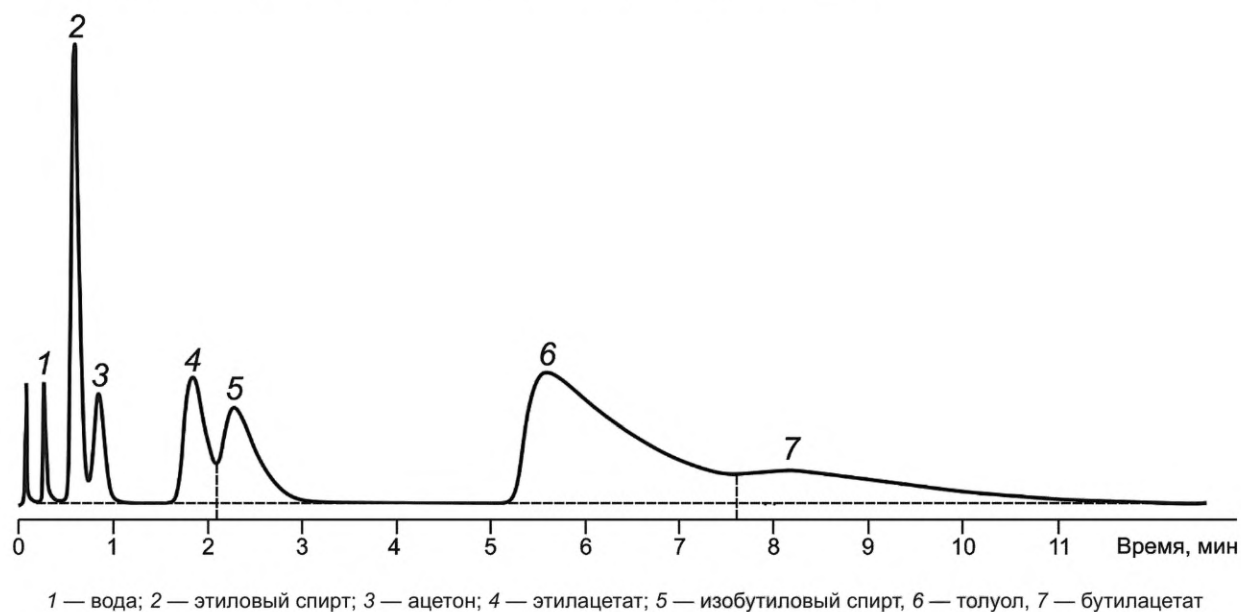
Рисунок Б.1 — Типовая хроматограмма растворителя марки 645
