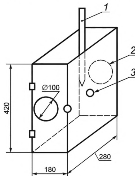
1 — пипетка; 2 — смотровое стекло; 3 — отверстие для зажима
