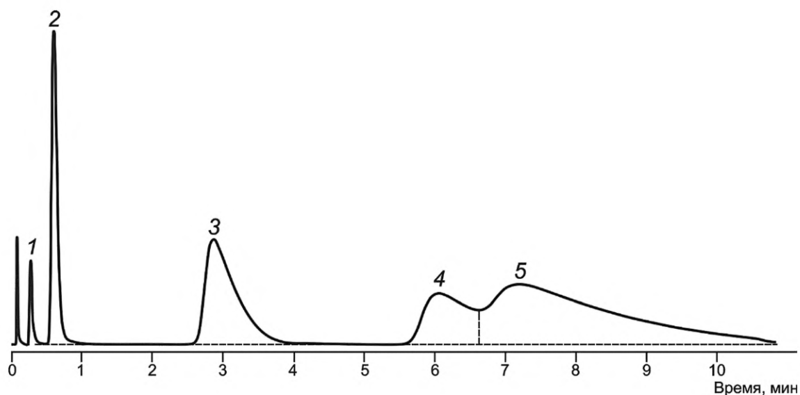
Рисунок Б.3 — Типовая хроматограмма растворителя марки 647
