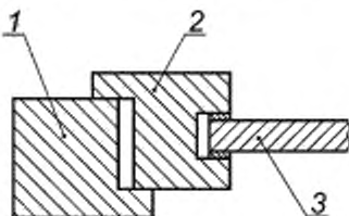
1 — коробка (неподвижная часть рамы); 2 — створка (подвижная часть рамы); 3 — остекление (одинарное, многослойное или стеклопакет)
