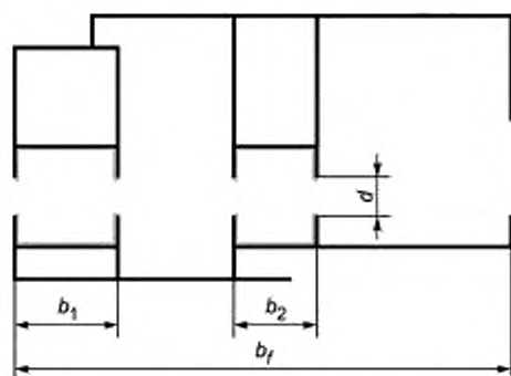
Рисунок F.6 — Поперечное сечение типа 2; теплопроводность материала термовставки менее 0,2 Вт/(м·К)
