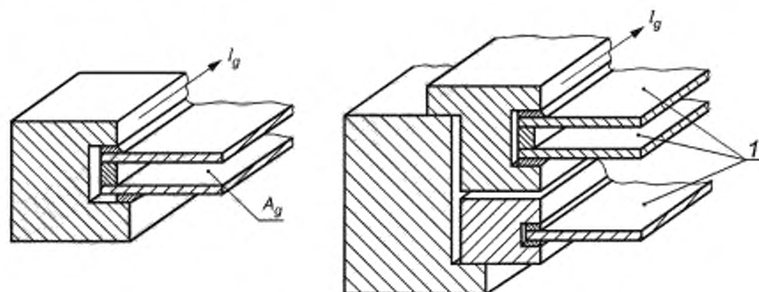
Рисунок 1 — Схема для определения площадей и периметра остекления
