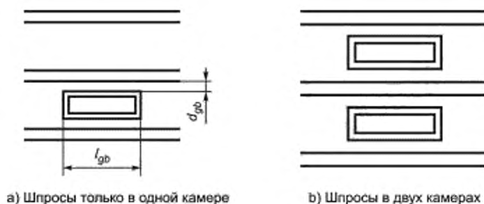
Рисунок G.3 — Схема двухкамерного стеклопакета со шпросами
