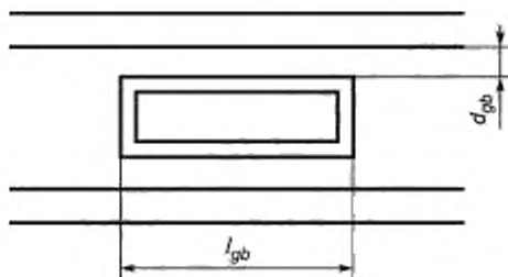
Рисунок G.2 — Схема однокамерного стеклопакета со шпросами
