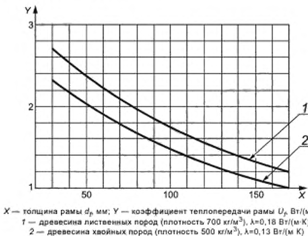
Рисунок F.2 — Коэффициент теплопередачи для деревянных и деревометаллических рам (см. рисунок F.3) в зависимости от их толщины d_F
