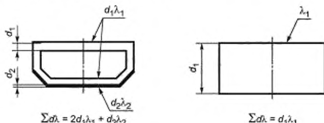
Рисунок G.1 — Примеры дистанционных рамок с улучшенной теплоизоляцией
