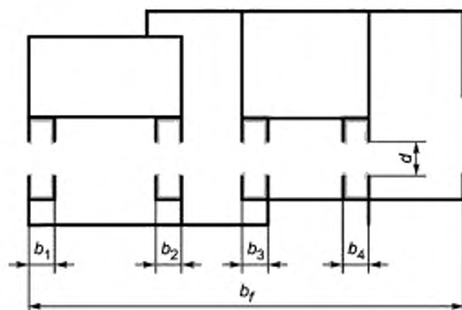
Рисунок F.5 — Поперечное сечение типа 1; теплопроводность материала термовставки менее 0,3 Вт/(м·К)
