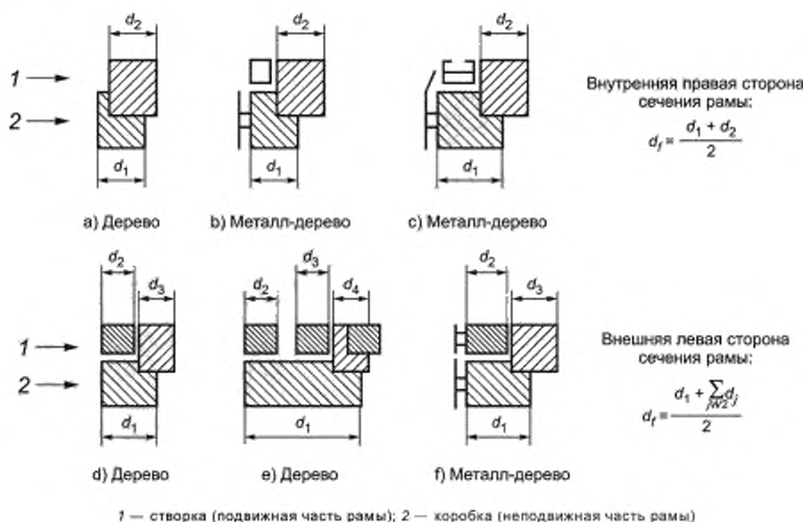
Рисунок F.3 — Расчет толщины рамы d_f для различных оконных систем
