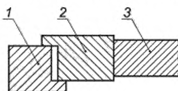
1 — коробка (неподвижная часть рамы); 2 — створка (подвижная часть рамы); 3 — непрозрачное заполнение
