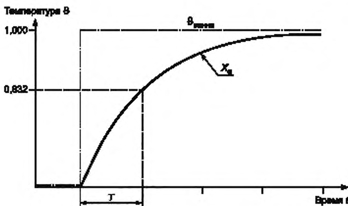
Рисунок ВВ.1 — Определение временного фактора в случае с внезапным изменением температуры
