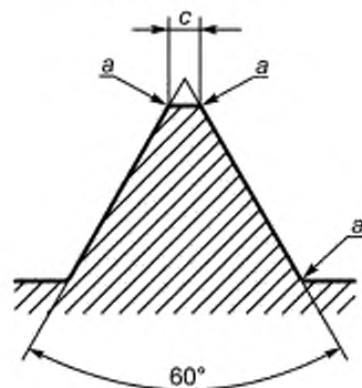
Профиль резьбы
