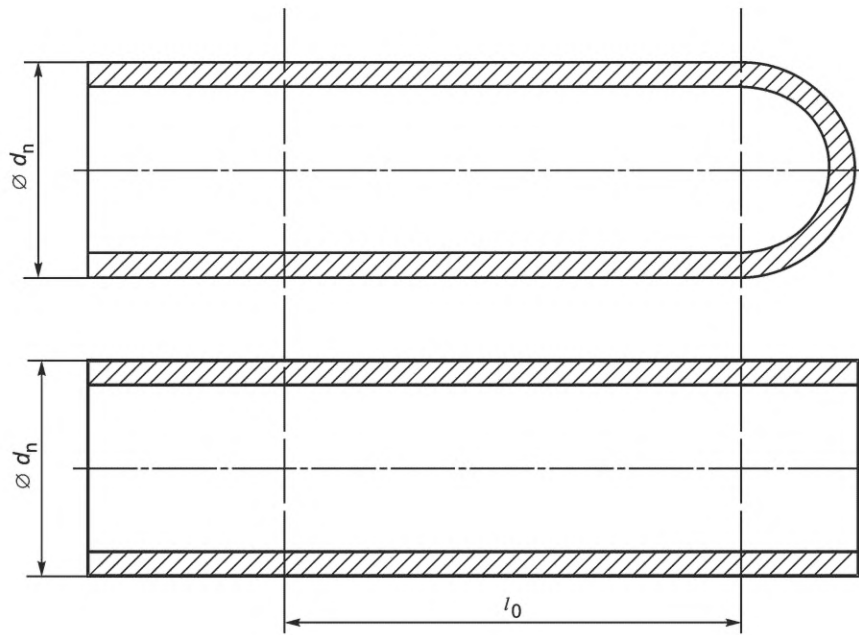
Рисунок 1 — Литьевые испытываемые образцы
