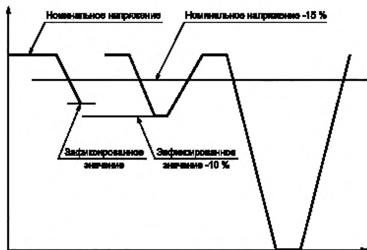
Рисунок Н.2 (пункт Н.26.5.4.2 в предыдущем издании) — Испытание изменения напряжения
