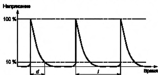
Рисунок 101 — Генерация импульсного искрового поджига
