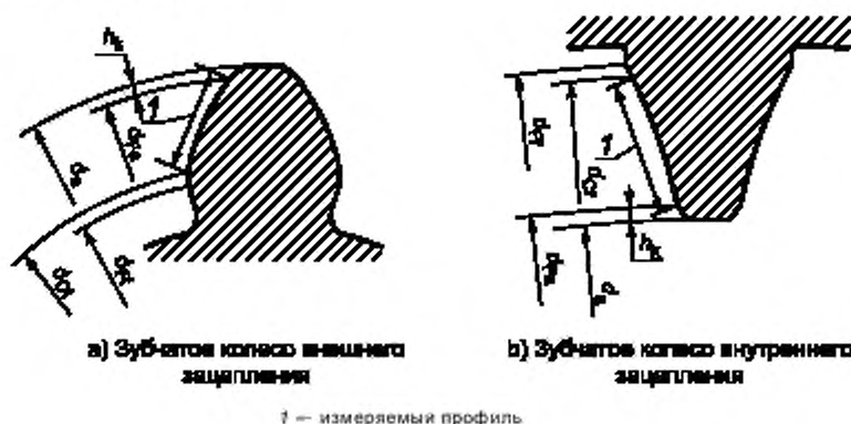
Рисунок 3 — Измеряемый профиль
