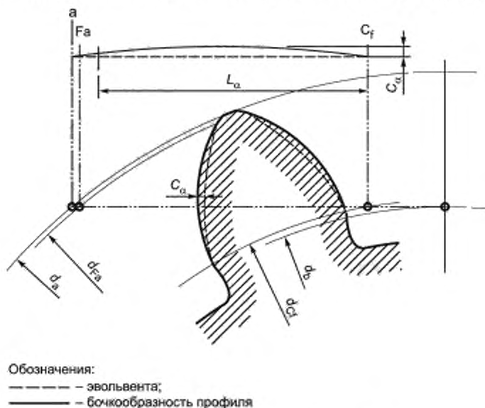
Рисунок В.1 — Бочкообразность профиля
