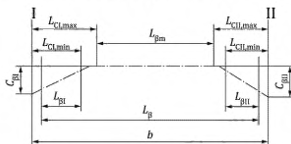
I — базовый торец; II — не базовый торец; C_{\beta I} — значение от среза торца; C_{\beta II} — значение от среза торца; L_{CI, \max} — максимальная длина от среза торца; L_{CI, \min} — минимальная длина от среза торца; L_{CII, \max} — максимальная длина от среза торца; L_{CII, \min} — минимальная длина от среза торца; L_{\beta I} — зона среза торца; L_{\beta II} — зона среза торца; L_{\beta m} — средняя зона направления линии зуба;
