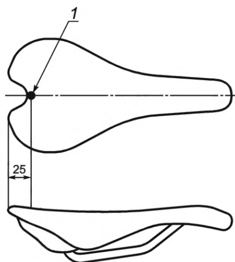
1 — точка нагружения
