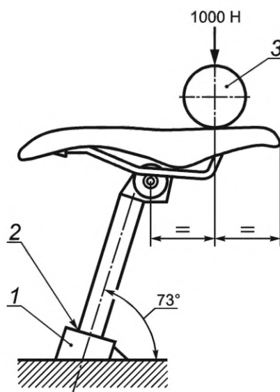
1 — жесткий зажим; 2 — отметка минимальной глубины погружения; 3 — проставка (длина — 300 мм, диаметр — 80 мм)
