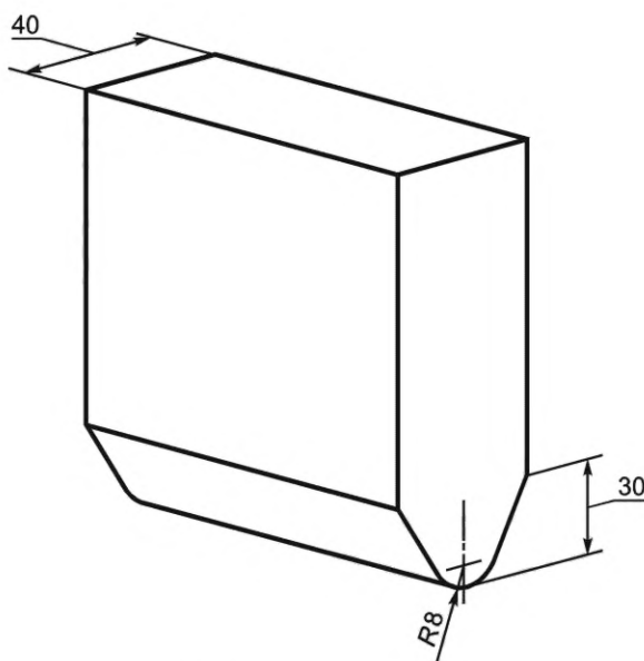
Рисунок 2 — Размеры ударника
