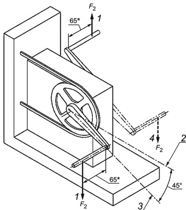
1 — повторяющиеся испытательные усилия; 2 — горизонтальная ось; 3 — ось шатуна; 4 — альтернативная схема расположения шатуна на неприводной стороне
