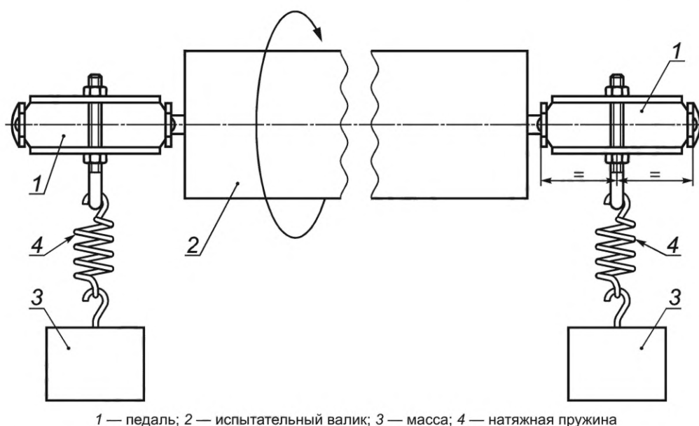
Рисунок 4 — Педаль/ось педали в сборе. Динамическое испытание на долговечность
