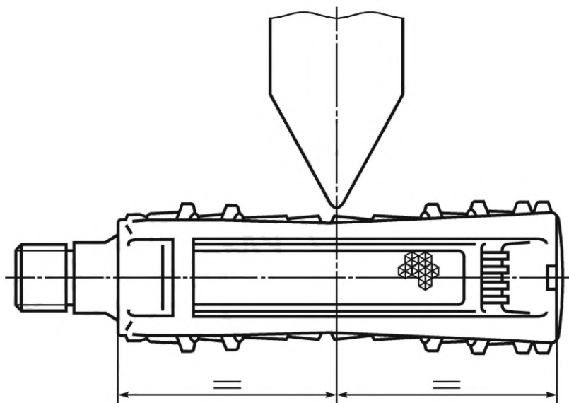
Рисунок 3 — Схема удара
