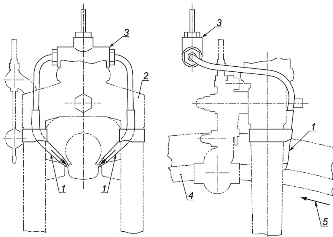
Рисунок 7 — Распылители воды для ободного тормоза (переднего)
