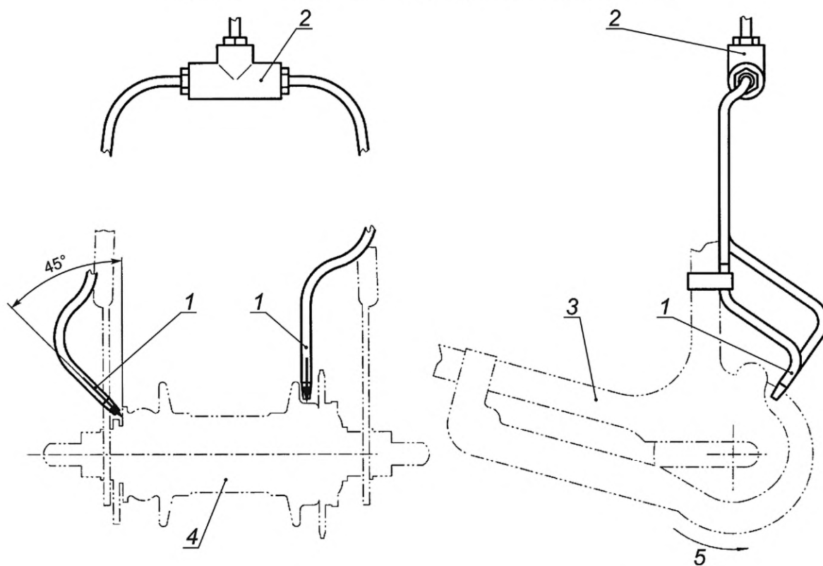
Рисунок 12 — Распылители воды для дискового тормоза (заднего)
