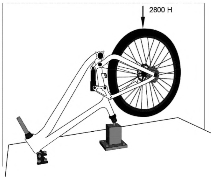
Рисунок С.1 — Примеры рам со встроенным упругим элементом. Испытание на зазор с шиной
