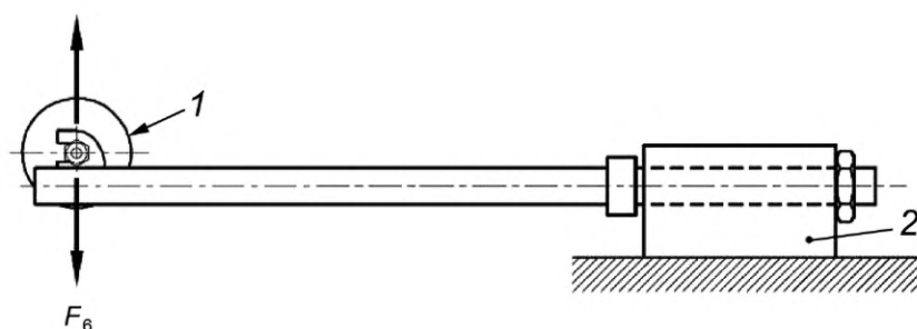
Рисунок 10 — Передняя вилка. Усталостное испытание на изгиб
