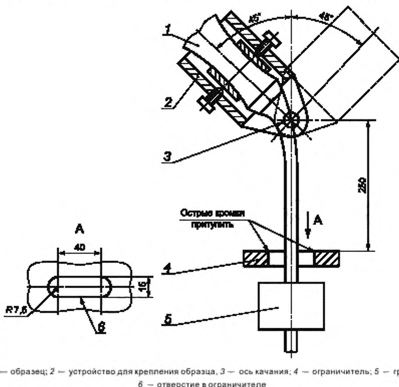
Рисунок 2 — Устройство для испытания светильника на изгиб
