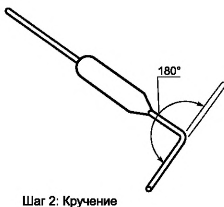
Рисунок 1 — Изгибающая/скручивающая сила
