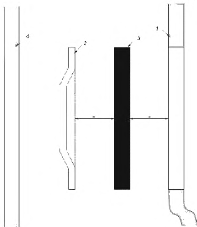
1 – дверь, люк или крышка; 2 – рельса для установки аппаратов и электрических устройств; 3 – резистор; 4 – задняя поверхность корпуса
