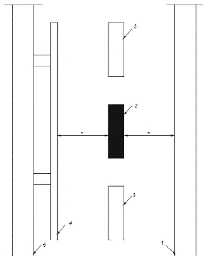
1 – дверь, люк или крышка; 2 – резистор; 3 – резисторы, если более одного; 4 – монтажная поверхность; 5 – задняя поверхность корпуса
