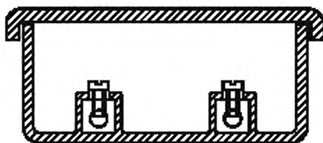
а — со встроенными зажимными компонентами
