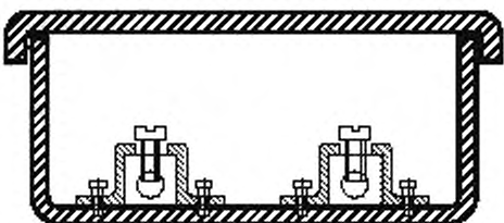
с — с условиями для вставки впоследствии оконечных или соединительных устройств
