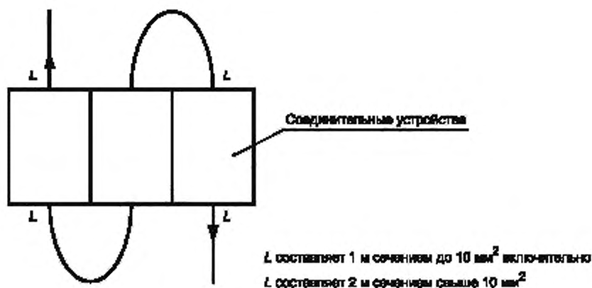
Рисунок 102 — Многопозиционное оконечное устройство
