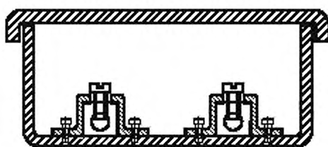
б — со вставленными выводами или соединительными устройствами
