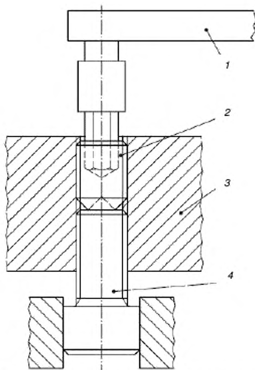
1 – ключ с регулируемым крутящим моментом; 2 – установочный винт для испытаний; 3 – контрольная плита: твердость не менее 50 HRC, допуск резьбы отверстия 5H (см. ISO 965-3); 4 – винт поддержки: твердость от 450 HV до 570 HV
