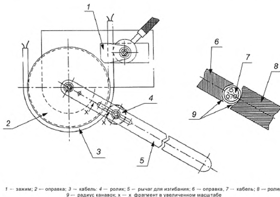
Рисунок 1 — Устройство для испытания на изгиб
