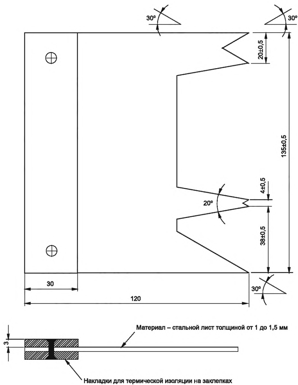
Рисунок 3 — Прибор для измерения высоты пламени
