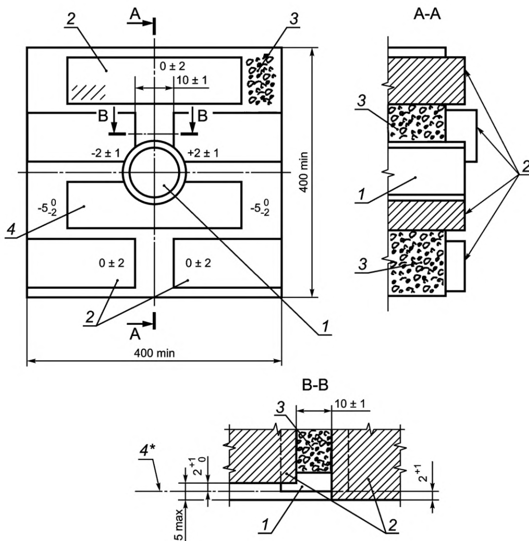
1 — коробка; 2 — кирпич; 3 — строительный раствор; 4 — контрольная поверхность
