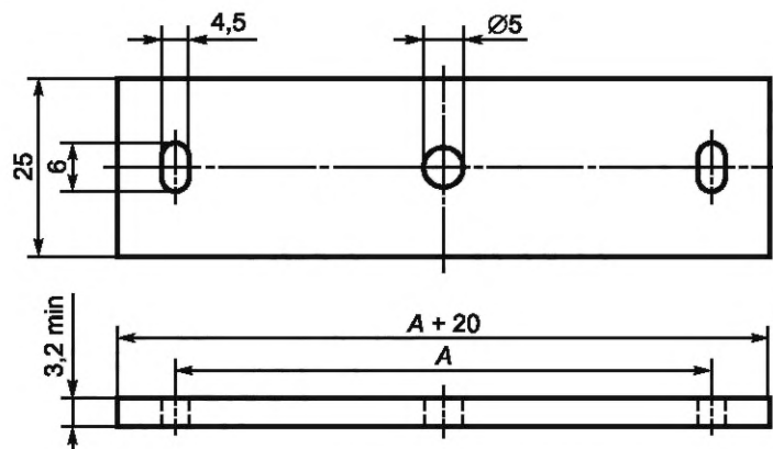
Рисунок 25 — Жесткая вставка
