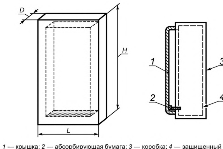
1 — крышка; 2 — абсорбирующая бумага; 3 — коробка; 4 — защищенный объем
