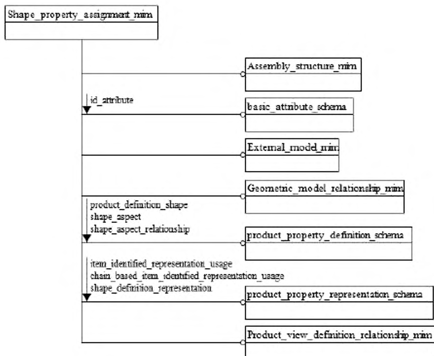
Рисунок D.1 – Представление ИММ на уровне схем в формате EXPRESS-G (диаграмма 1 из 1)
