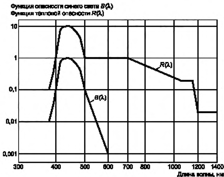
Рисунок 6 — Функция тепловой опасности для сетчатки R(\lambda) и функция опасности синего света для сетчатки B(\lambda)
