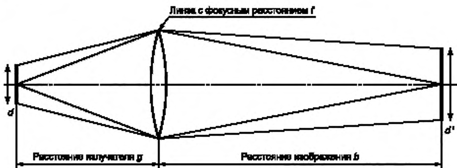
Рисунок 9 — Определение углового размера источника
