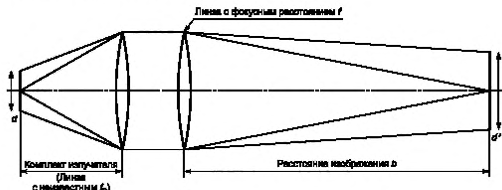
Рисунок 10 — Определение углового размера источника
