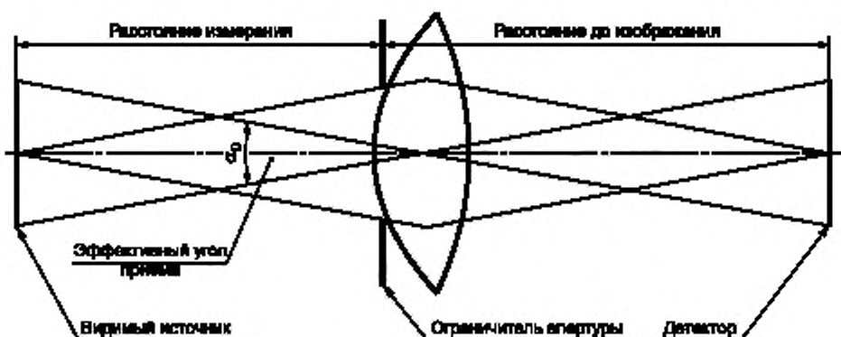
Рисунок 8 — Условия измерения для определения интегрированной по времени энергетической яркости
