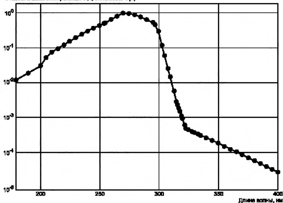
Относительная спектральная эффективность S(\lambda)
