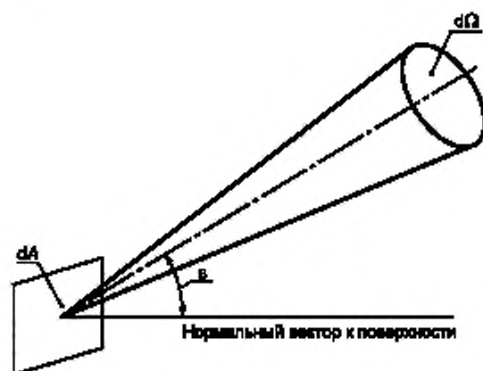
Рисунок 2 — Определение энергетической яркости
