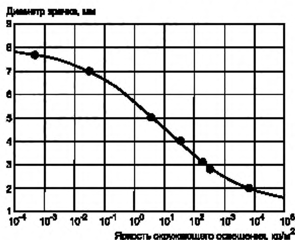
Рисунок 4 — Зависимость диаметра зрачка от яркости наблюдаемого поля в соответствии с [5].
