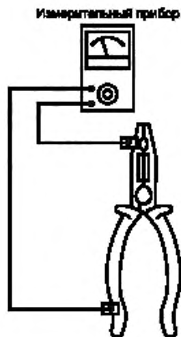
Рисунок 16 — Измерение сопротивления ручного инструмента
