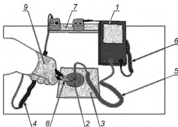
а) Сопротивление инструмента к системе заземления
