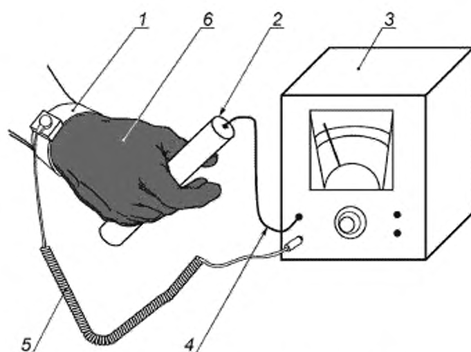
а) Использование омметра для испытаний
