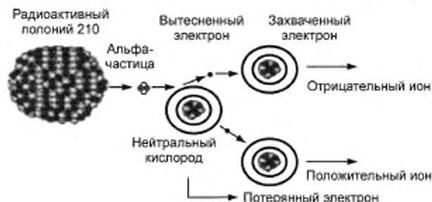
Рисунок 6 — Ионизация альфа-излучением
