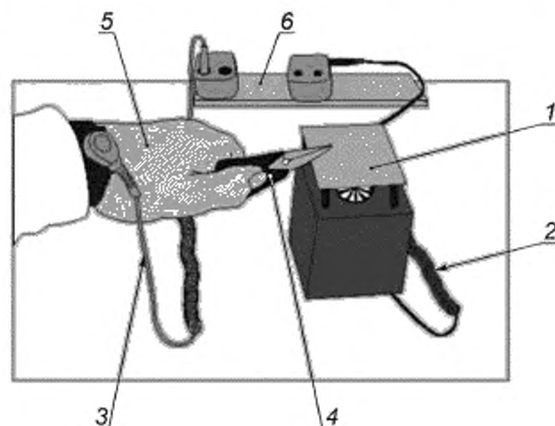
а) Измерение стекания заряда с инструмента
