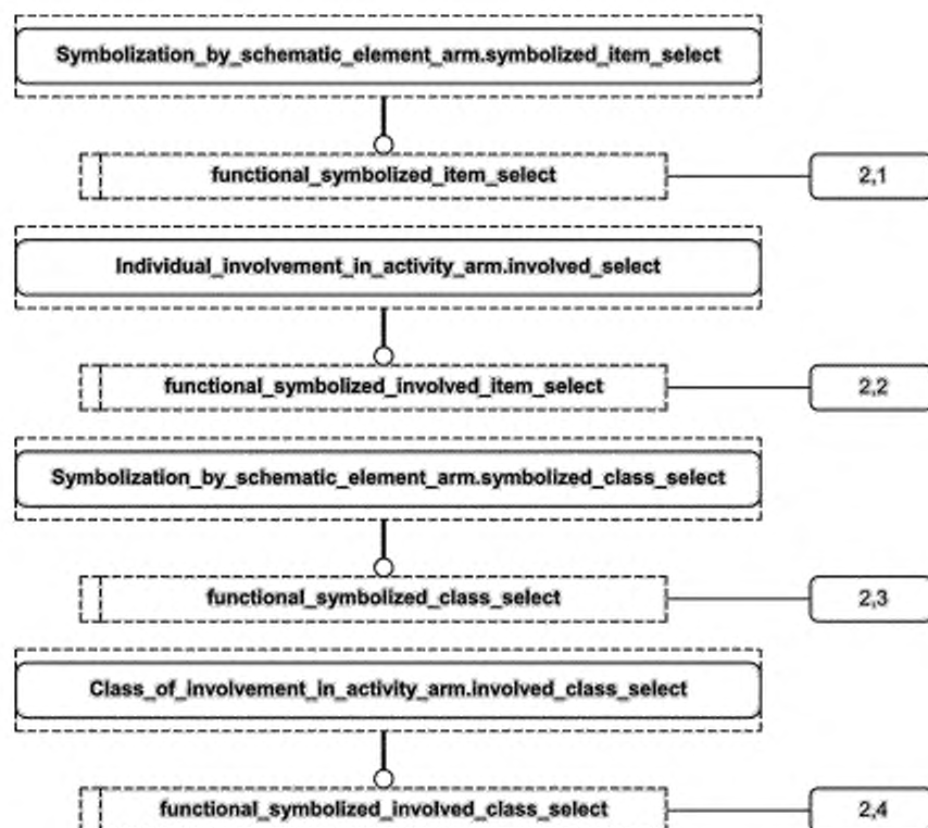
Рисунок С.2 — Представление ПЗМ на уровне объектов в формате EXPRESS-G (диаграмма 1 из 5)
