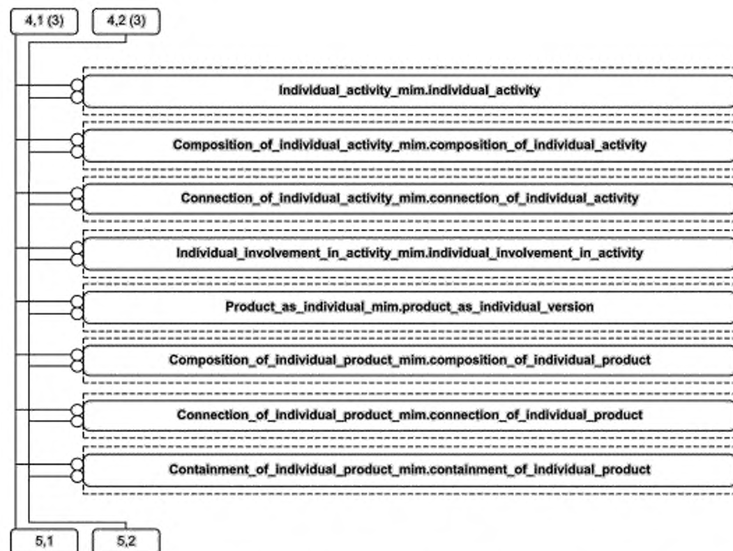
Рисунок D.5 — Представление ИММ на уровне объектов в формате EXPRESS-G (диаграмма 4 из 5)
