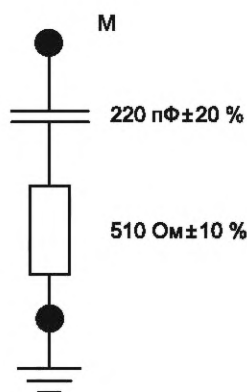
Рисунок 2 — Эквивалент руки, RC-элемент
