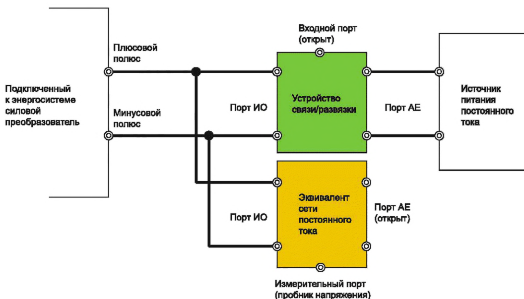
Рисунок 7 — Типовая установка для измерения кондуктивных помех на низковольтных портах электропитания постоянного тока с эквивалентом сети постоянного тока (DC-AN), используемым в качестве оконечного устройства и пробника напряжения
