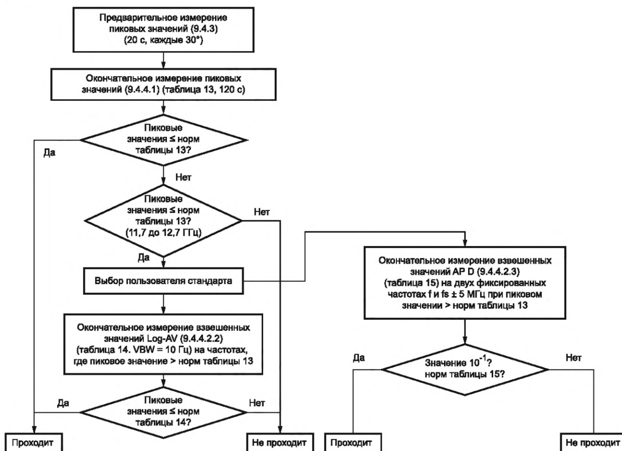
Рисунок 12 — Алгоритм для проведения измерения излучаемых радиопомех в диапазоне частот от 1 до 18 ГГц оборудования группы 2, работающего на частотах выше 400 МГц
