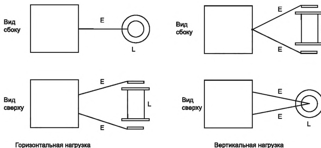
Рисунок 5 — Взаимное расположение медицинского оборудования (конденсаторного типа) и эквивалента нагрузки
