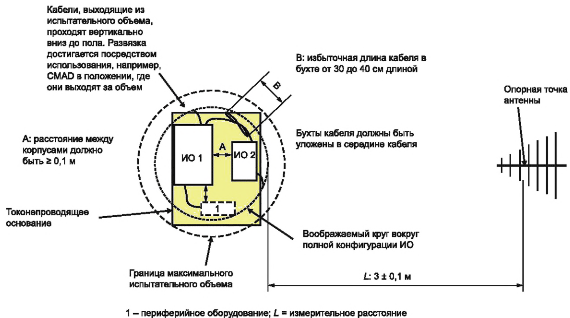
Рисунок 3а — Вид сверху
