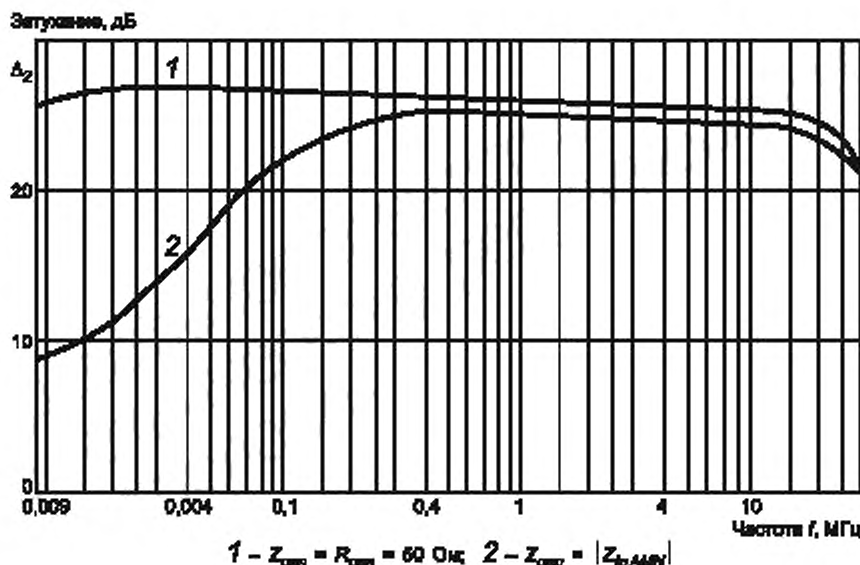
Рисунок А.5 — Затухание фильтра AMN
