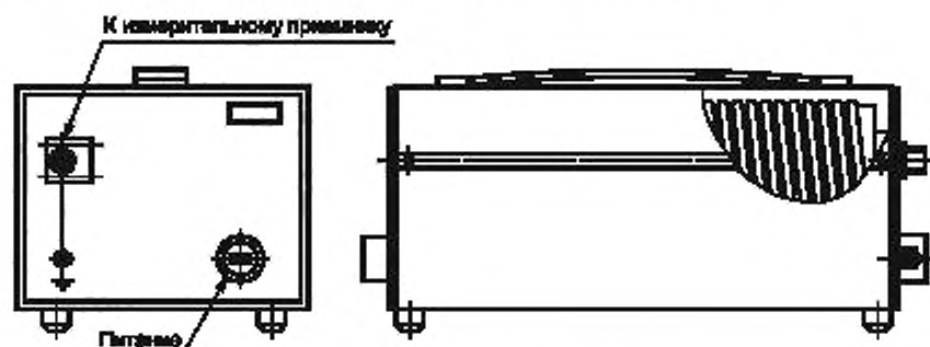
Рисунок A.4 — Общий вид AMN
