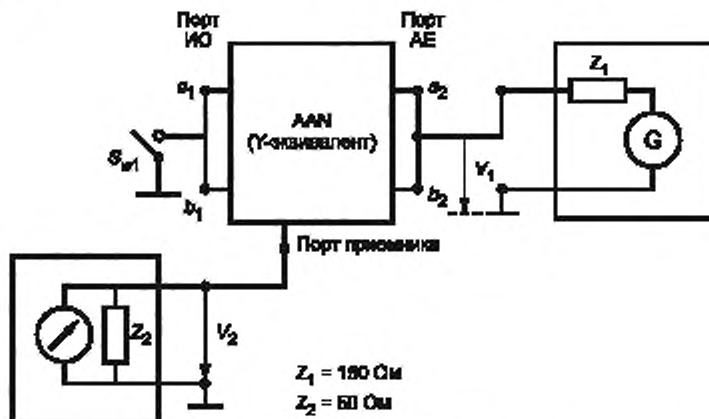
Рисунок Е.5 — Измерения LCL асимметричного эквивалента сети (AAN) с помощью пробника LCL
