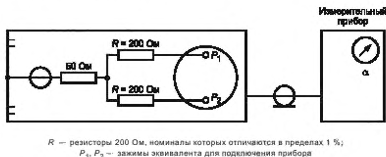
Рисунок 4 — Метод проверки симметрии схемы измерения симметричных напряжений
