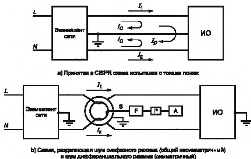
Рисунок В.4 — Испытательная установка для измерения тока с использованием AMN
