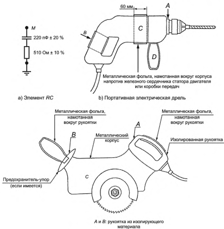
Рисунок 11 — Применение эквивалента руки
