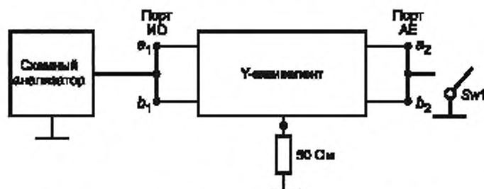
Рисунок Е.1 — Пример T -эквивалента сети для одной пары проводов
