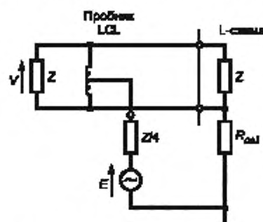
Рисунок Е.3 — Схема для проверки пробника LCL
