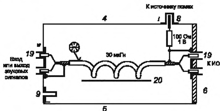
4—9 — см. устройство типа А; 19 — розетки DIN или с прижимными контактами; 20 — индуктивность 30 мкГн; Сердечник: одно ферритовое кольцо, материал типа 4С6, \varnothing 36 \text{ мм} \times \varnothing 23 \text{ мм} \times 15 \text{ мм} . Обмотка: 14 витков экранированной скрученной пары: внешний диаметр изоляции кабеля 2,8 мм. Монтаж катушки индуктивности: см. устройство типа А.
