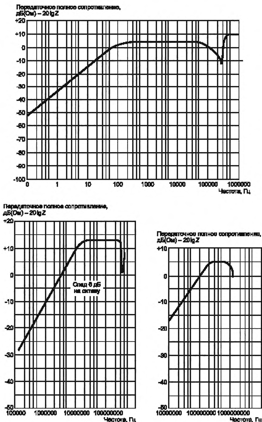
Рисунок В.3 — Передаточное полное сопротивление типовых токоъемников
