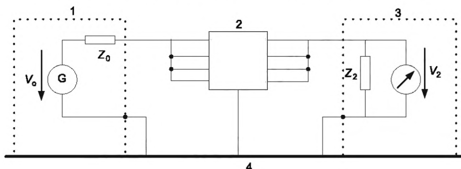
1 — генератор сигналов; 2 — фильтрующее устройство для обеспечения электромагнитной совместимости (испытуемое оборудование); 3 — измерительный приемник; 4 — опорный потенциал (металлическая пластина заземления); V_0 — напряжение холостого хода генератора; V_2 — выходное напряжение; Z_0 — полное сопротивление генератора; Z_2 — полное сопротивление приемника
