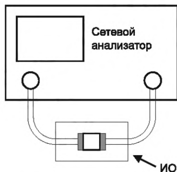
Рисунок 15 — Схема измерения S-параметров двух портов
