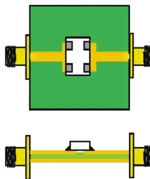
б) испытательное устройство со встроенным СД
