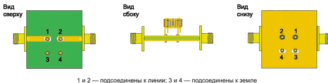
Рисунок G.7 — Испытательное устройство для оборудования с выводами
