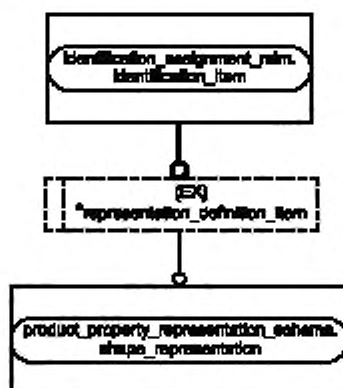
Рисунок D.2 — Представление IMM на уровне объектов в формате EXPRESS-G
