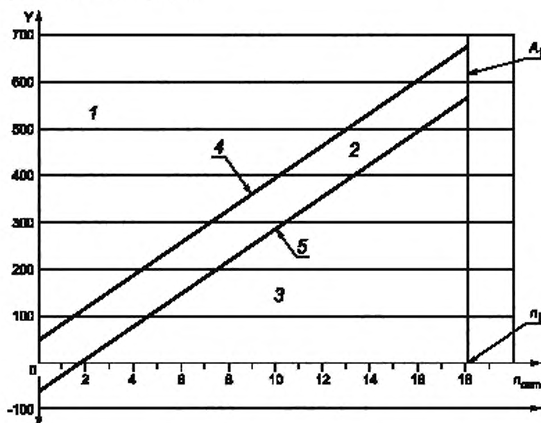
Рисунок 1 — Приемочная карта для последовательного плана выборочного контроля и единственной границы поля допуска
