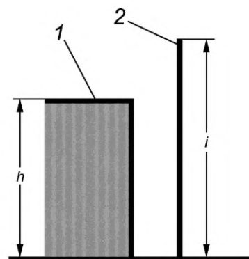
Рисунок 2б — Положение индикатора для h < 2 м
