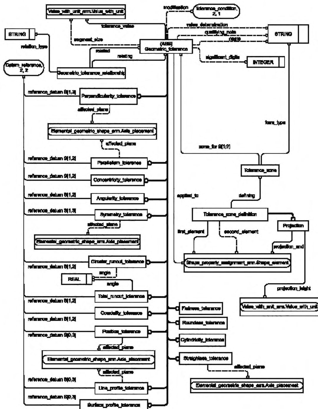
Рисунок С.2 — Представление ПЗМ на уровне объектов в формате EXPRESS-G (диаграмма 1 из 2)
