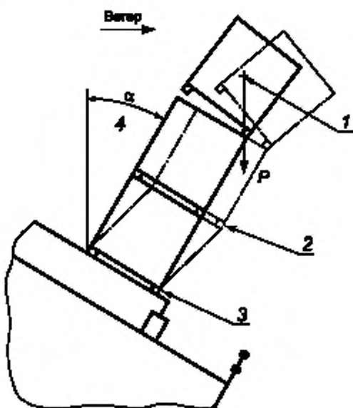
1 — опрокидывающая сила; 2 — сила перекоса; 3 — сила скольжения; 4 — качка
