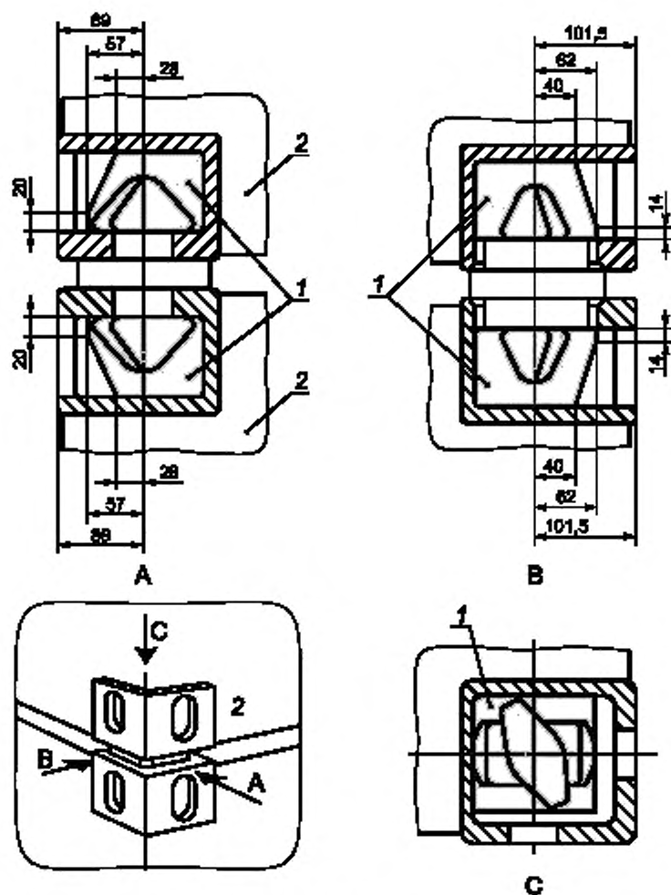
Рисунок D.7 — Ограниченная часть полости углового фитинга
