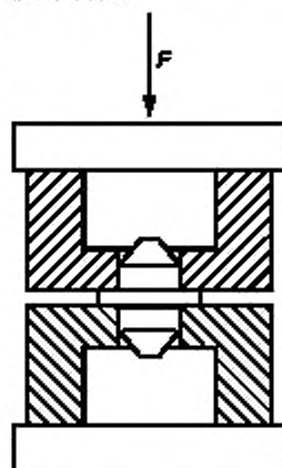
F — испытательная сила
