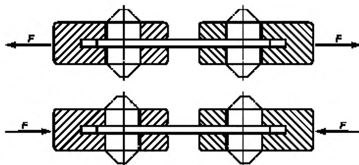
Рисунок С.9 — Испытание на растяжение и сжатие
