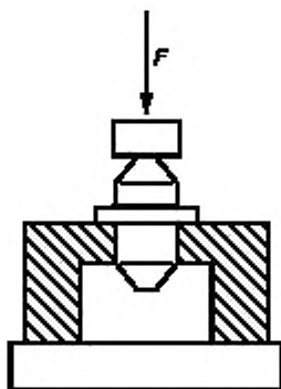
F — испытательная сила
