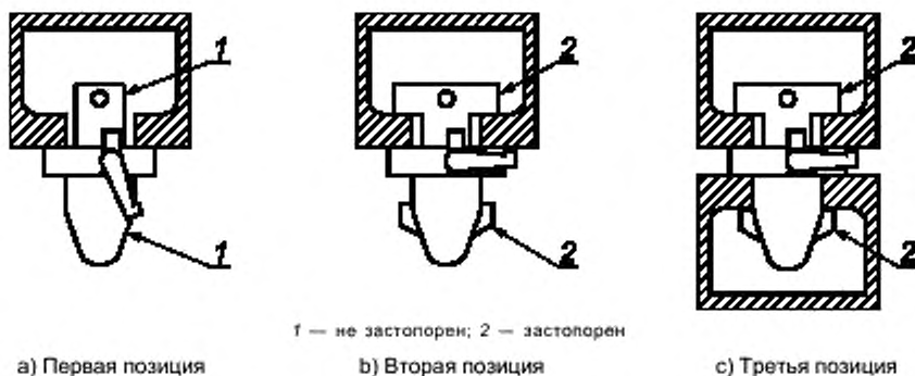
Рисунок В.2 — Полуавтоматический стопор, установленный в нижний угловой фитинг
