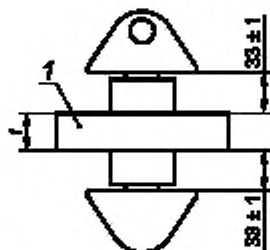
Рисунок А.9 — Расстояние между верхним и нижним конусами
