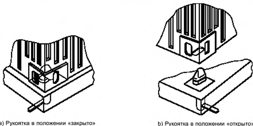
Рисунок 26 — Стопоры с поворотной головкой на несущей платформе
