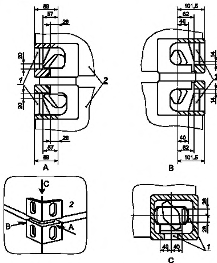
Рисунок А.5 — Ограниченная часть полости углового фитинга
