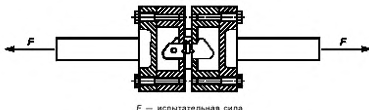
Рисунок В.9 — Испытание стопора на растяжение
