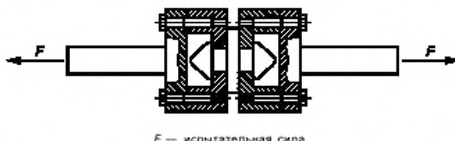
Рисунок A.10 — Испытание стопора (твистлока) на растяжение
