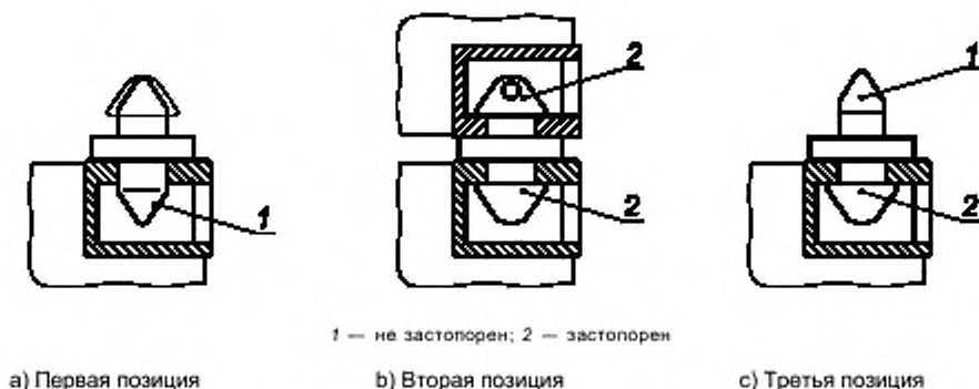
Рисунок А.3 — Полуавтоматический стопор, установленный в нижний угловой фитинг
