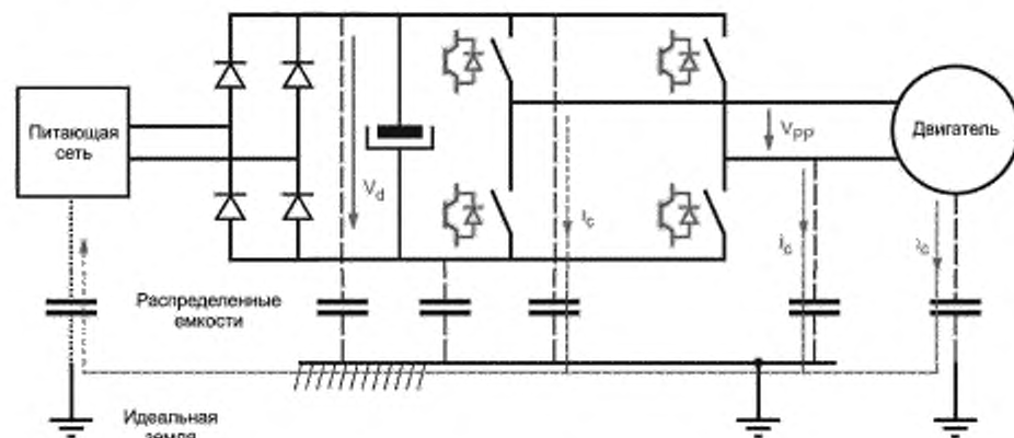
Рисунок A.5 — Пример распределенной емкости установки на землю
