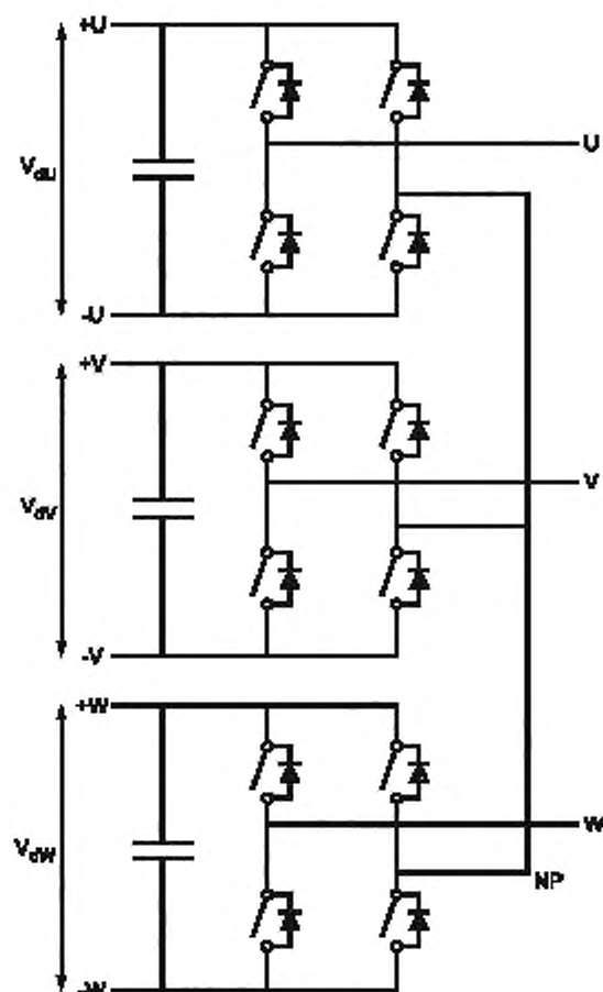
Рисунок 30 — Топология трехуровневого инвертора напряжения (много звеньев постоянного тока). n_{\text{dcmult}} = 1 . Напряжения V_{dx} остаются неизменными
