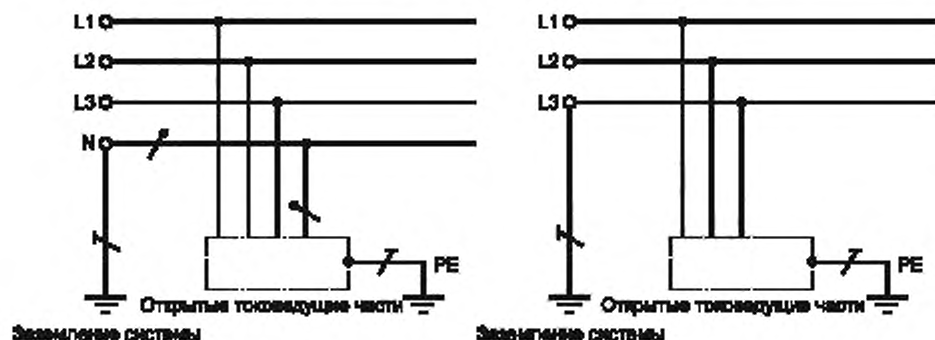
Рисунок A.3 — Система питания TT
