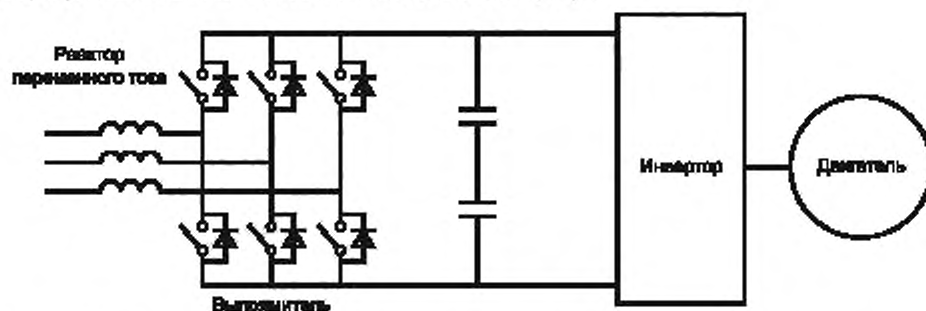
Рисунок 24 — Типичная схема преобразования напряжения с трехфазным активным выпрямителем
