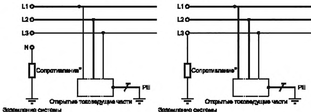
Рисунок A.4 — Система питания IT
