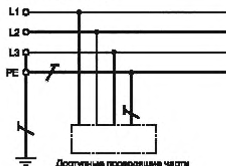
Заземленная система
