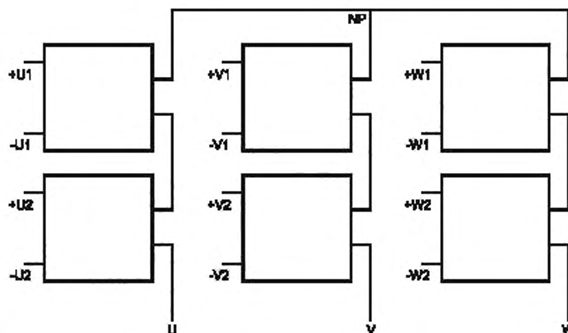
Рисунок 31 — Топология N-уровневого инвертора напряжения (много звеньев постоянного тока), n_{dcmult} = 2
