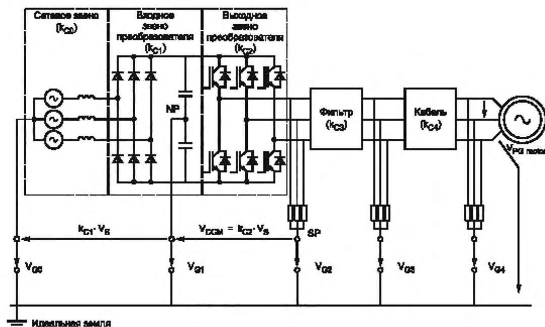
Рисунок 39 — Эквивалентная цепь для синфазной модели
