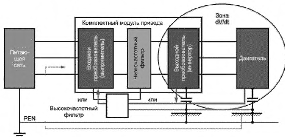
Рисунок A.7 — Пример протекания токов утечки при системе заземления IT
