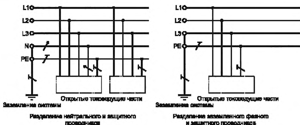
Рисунок A.1 — Система питания TN-S
