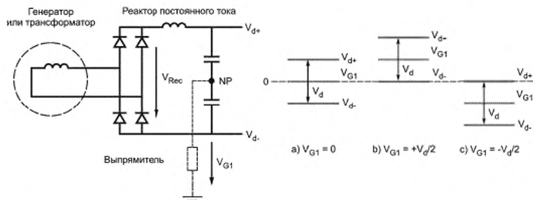
Рисунок 16 — Типичная конфигурация инвертора напряжения с неуправляемым однофазным выпрямителем. L 1 и L 2 для систем питания IT
