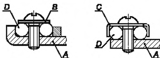
A — зафиксированная часть; B — шайба или прижимная пластина; C — устройство, ограничивающее распушивание проводника. D — пространство для укладки проводника
