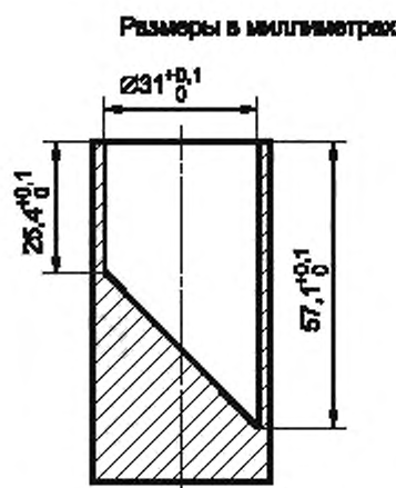
Рисунок 16 — Цилиндр для проверки размеров небольших компонентов
