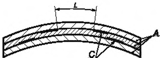
L — расстояние между соседними проводниками; A — слой тонкопленочного материала, например ленты полиэфирной пленки; C — проводники
