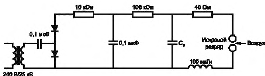
Рисунок А.1 — Пример простой электрической схемы, моделирующей работу преобразователя
