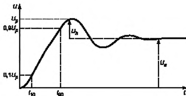
Рисунок 1 — Параметры импульса напряжения
