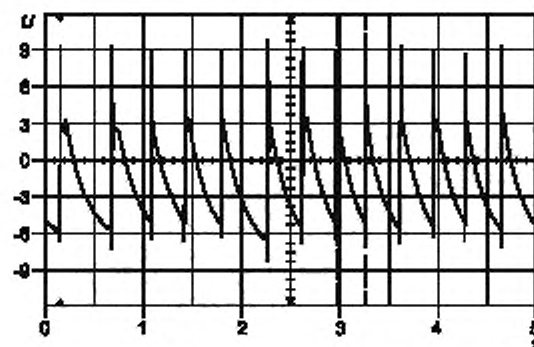
Рисунок А.2 — Типичные осциллограммы напряжения, генерируемого искровым разрядником ( U , кВ; t , мс)
