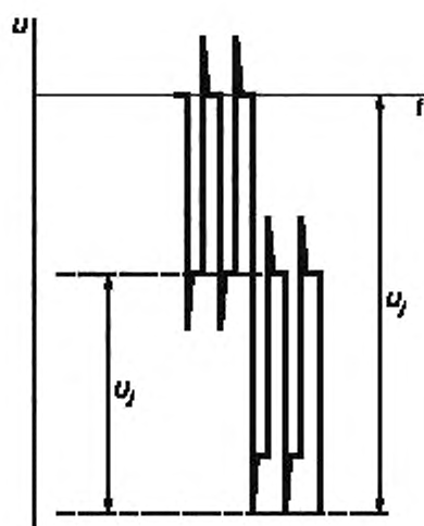
Рисунок 3 — Возможный скачок напряжения U_j на зажимах машины, связанный с типом преобразователя
