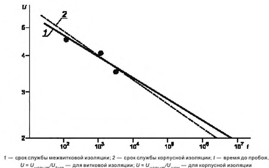
Рисунок 6 — Срок службы межвитковой и корпусной изоляции
