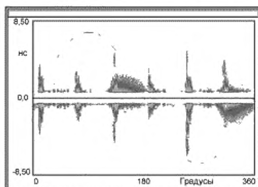
Рисунок D.1 — Диаграмма без маскировки
