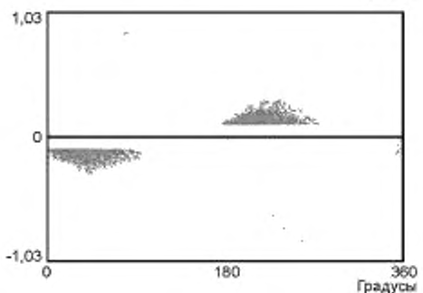
Разряды во внутренних полостях Разряды во внутренних полостях основной изоляции
