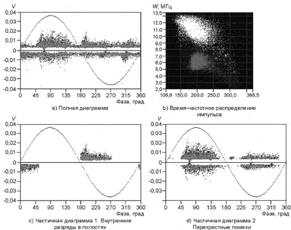
Рисунок D.5 — Пример выделения перекрестных помех
