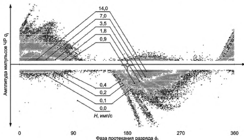
Рисунок 4 — Пример \phi - q - n диаграммы рассеяния импульсов ЧР на объекте, представленном на рисунке 5б.
