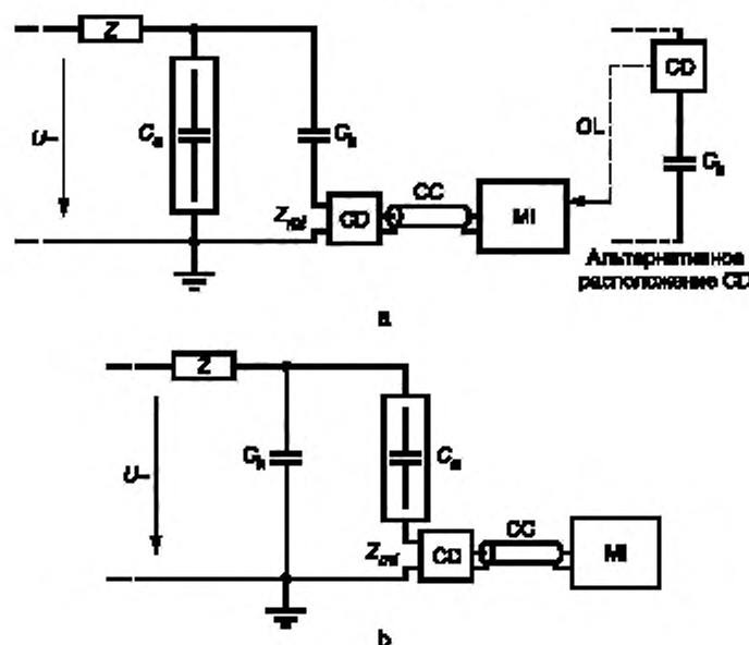
а — соединительное звено последовательно с соединительным конденсатором, б — соединительное звено последовательно с испытуемым объектом, U — высоковольтный источник; Z_{in} — входное сопротивление измерительной системы; CC — соединительный кабель; OL — оптическая линия связи; C_n — испытуемый объект, C_k — соединительный конденсатор; CD — соединительное звено; MI — измерительный прибор; Z — фильтр
