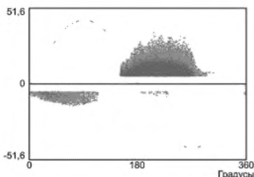
Рисунок Е.1 — Примеры диаграмм ЧР
