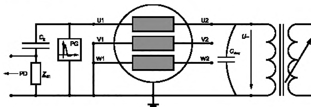
U — высоковольтный источник; Z_m — измерительное сопротивление; C_k — емкость соединительного конденсатора; C_{stray} — паразитная емкость; PG — генератор импульсов по IEC 60270; PD — частичный разряд
