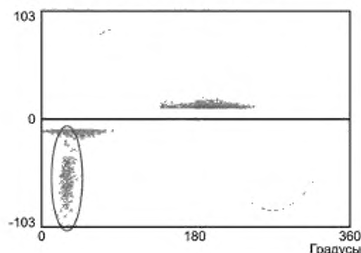
Разряды в лобовых частях обмоток Поверхностные разряды в лобовых частях в результате загрязнения поверхности изоляция-воздух
