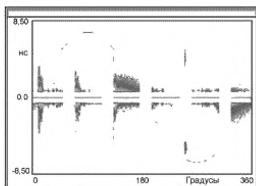
Рисунок D.2 — Диаграмма с маскировкой
