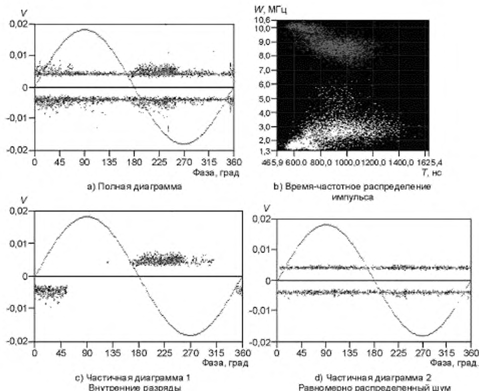
Рисунок D.4 — Пример шумоподавления
