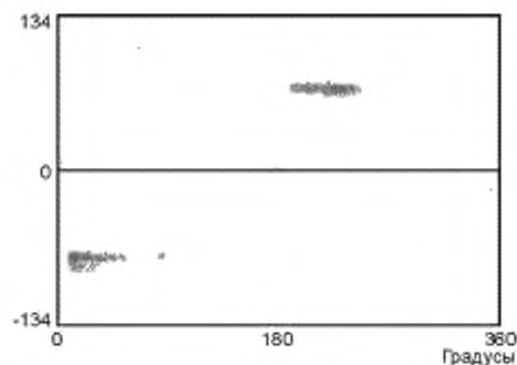
Разряды в лобовых частях обмоток Разряды в зазорах между проводниками лобовых частей или между стержнями и арматурой сердечника
