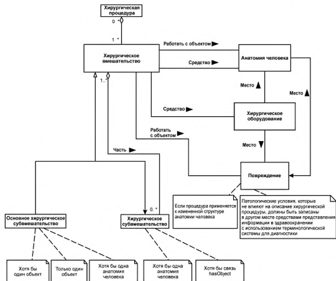
Рисунок 1 — UML диаграмма
