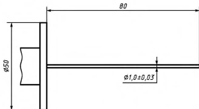
Рисунок 2 - Испытательный щуп
