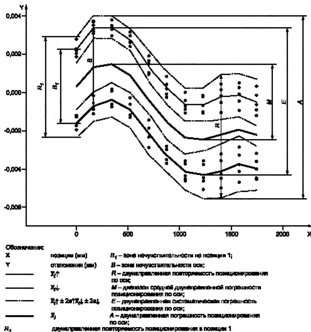
Рисунок 2 — Двунаправленная погрешность и повторяемость позиционирования
