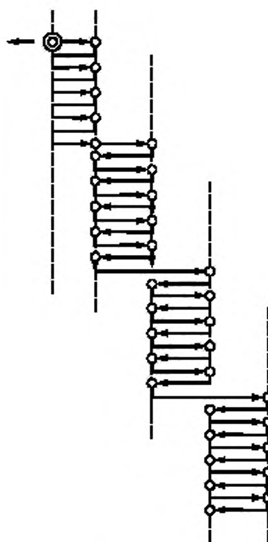
Рисунок В.1 — Ступенчатый цикл
