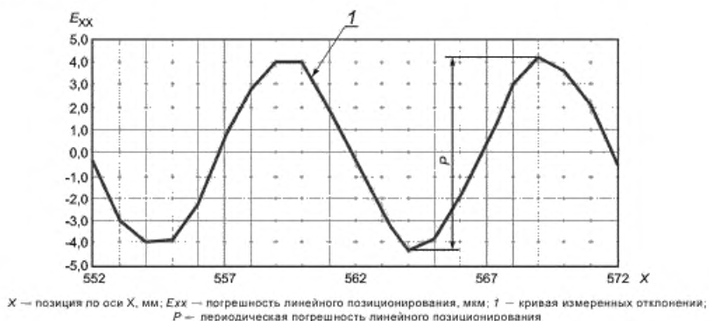
Рисунок С.1 — Пример периодической погрешности линейного позиционирования для оси X с шариковым винтом с шагом 10 мм, электродвигателем с прямой передачей вращения и угловым преобразователем на валу электродвигателя
