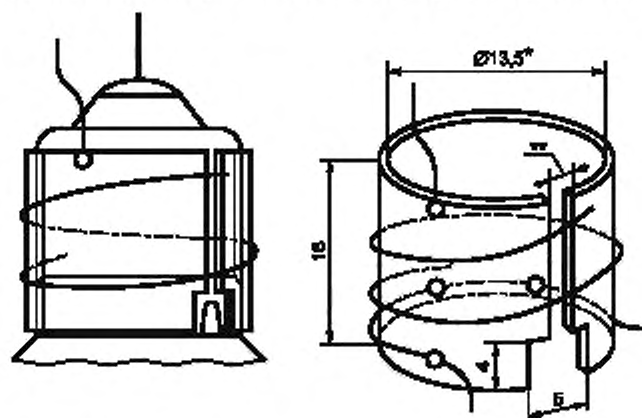
Приблизительные размеры испытательного патрона для цоколя E14/20, мм
