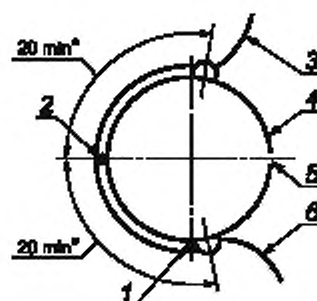
Положение испытательного патрона и термопреобразователя
