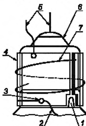
Испытательный патрон для ламп с резьбовым цоколем
