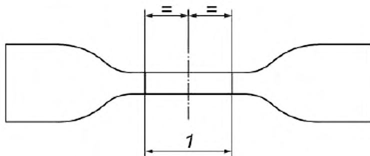
Рисунок 2 — Форма образца лопатки
