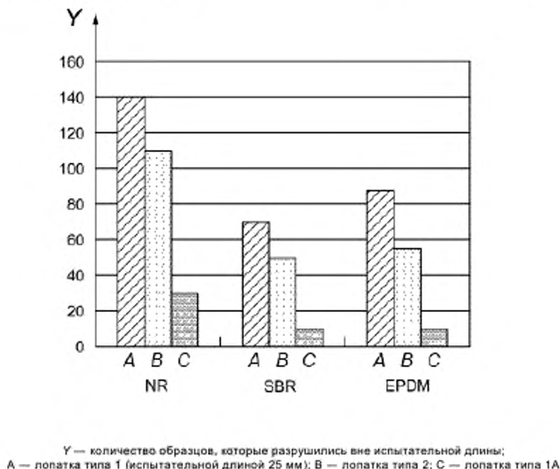
Р и с у н о к С.1 — Количество образцов, которые разрушились вне испытательной длины (первая ИТР — было испытано 230 образца каждого типа)
