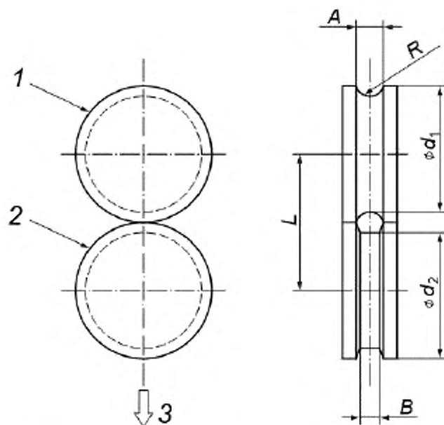
1 — свободно вращающийся шкив; 2 — неподвижный приводной шкив; 3 — направление растяжения
