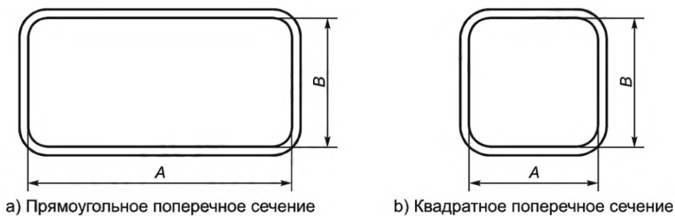
Рисунок 2 — Прямоугольные банки
