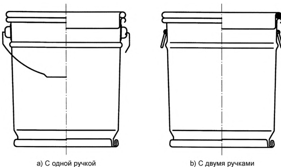
Рисунок 2 — Ведро
