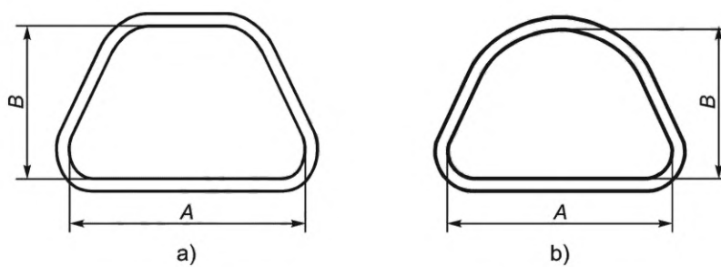
Рисунок 13 — Трапецевидные банки
