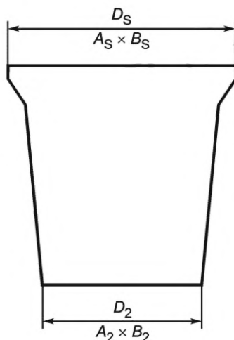
Рисунок 22 — Примеры обозначения банок общего назначения
