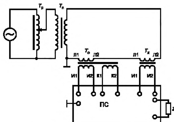
\sim — сеть (генератор); T_p — регулирующее устройство (автотрансформатор); T_n — понижающий силовой трансформатор; T_n — рабочий эталон; T_x — поверяемый трансформатор тока; L_1, L_2 — контактные зажимы первичной обмотки; I_1, I_2 — контактные зажимы вторичной обмотки; K_1, K_2 — контактные зажимы дополнительной вторичной обмотки; Z — нагрузка; ПС — прибор сравнения типа КТ-01
