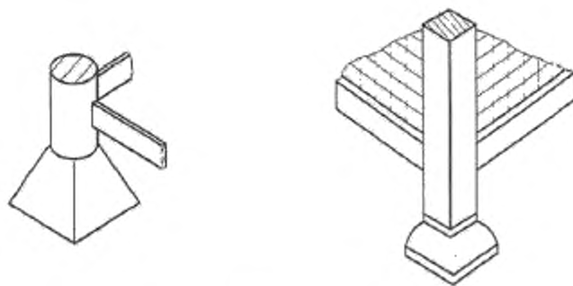
Рисунок 59 – Чашечная опора
