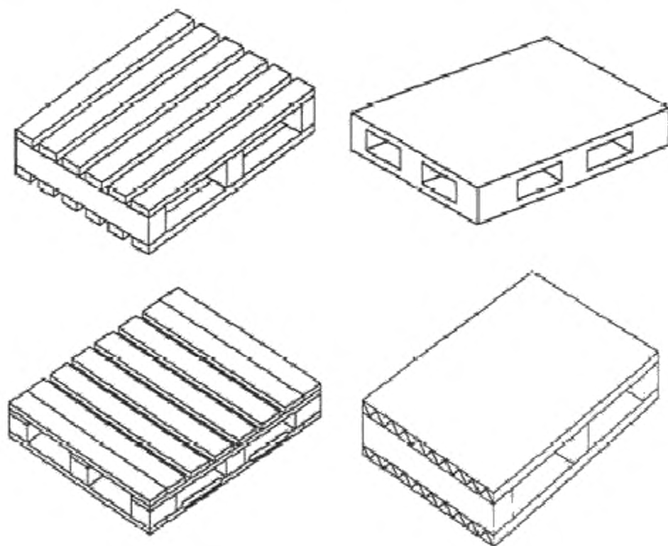
Рисунок 7 -- Необратимые поддоны
