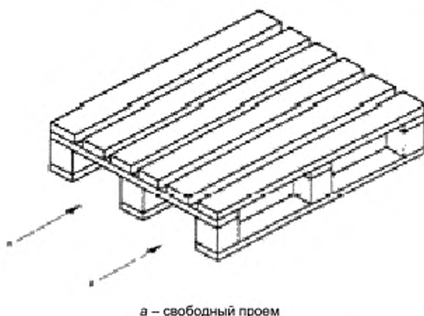
Рисунок 43 – Свободный проем поддона
