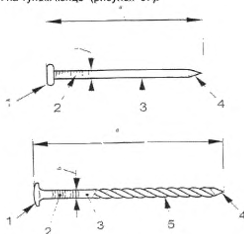
a — длина; b — диаметр 1 — головка; 2 — насечки в виде небольших канавок; 3 — гладкая поверхность гвоздя; 4 — острие; 5 — винтовая часть
