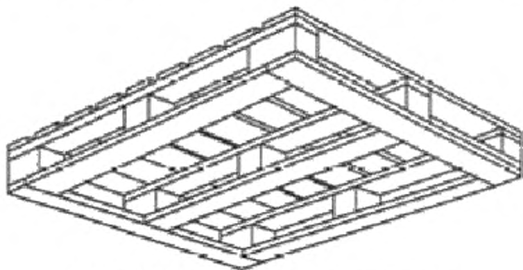
Рисунок 13 — Поддон с нижним настилом по периметру
