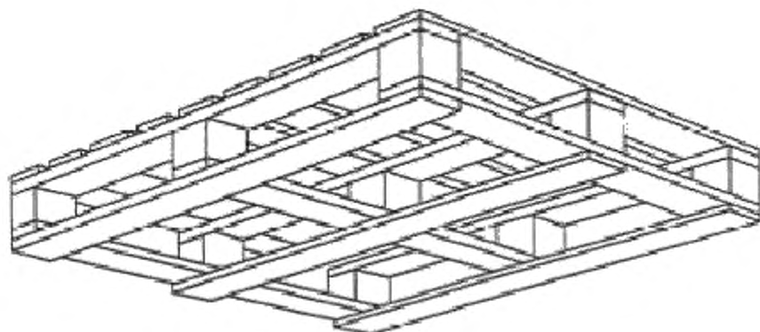
Рисунок 11 – Упрочненный поддон
