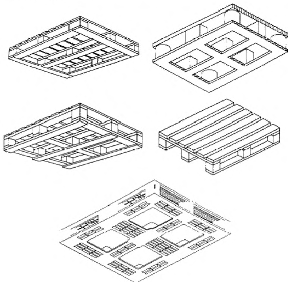
Рисунок 41 – Просветы поддонов
