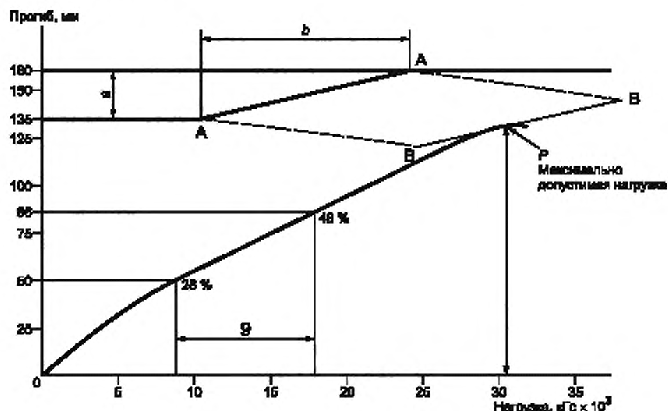
Рисунок 2 — Пример определения максимально допустимой нагрузки
