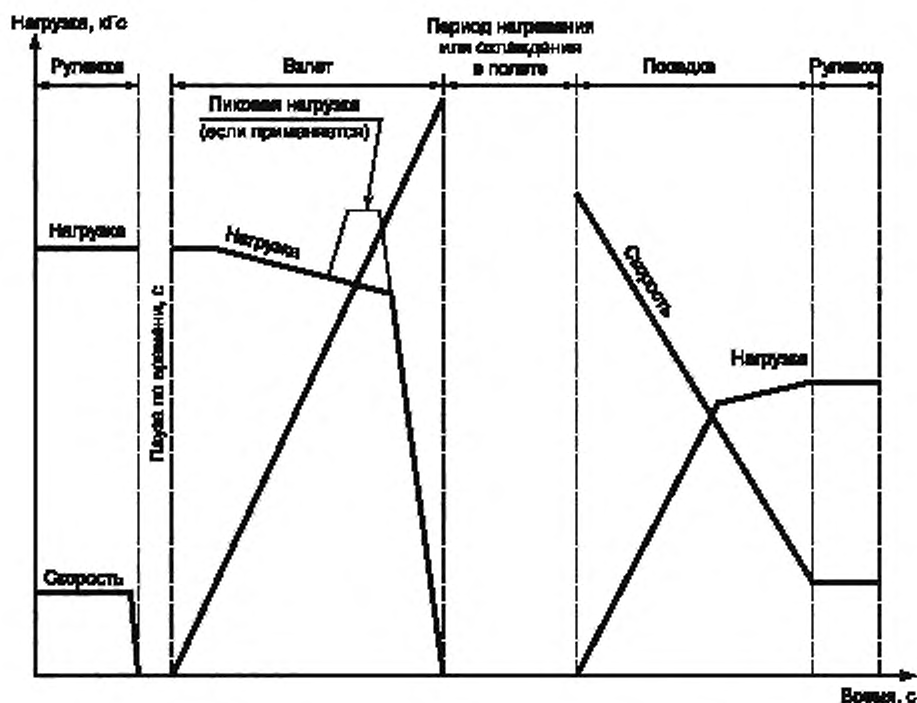
Рисунок 5 — Последовательность испытательного цикла — общий цикл
