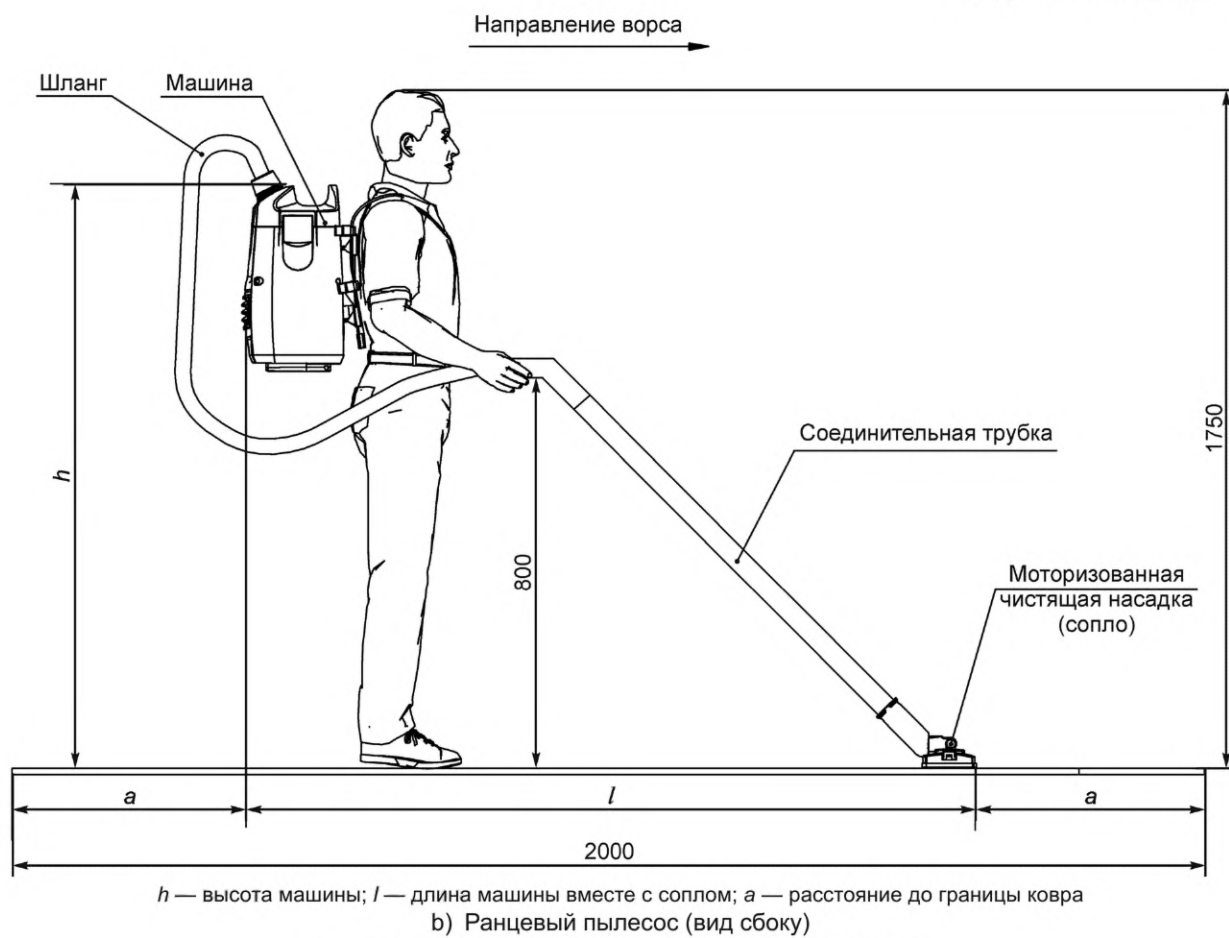
Рисунок EE.3 — Расположение ранцевых пылесосов
