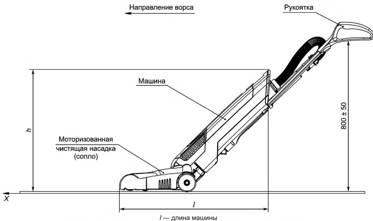
б) Машина с чистящей насадкой, оснащенная шлангом (вид сбоку)
