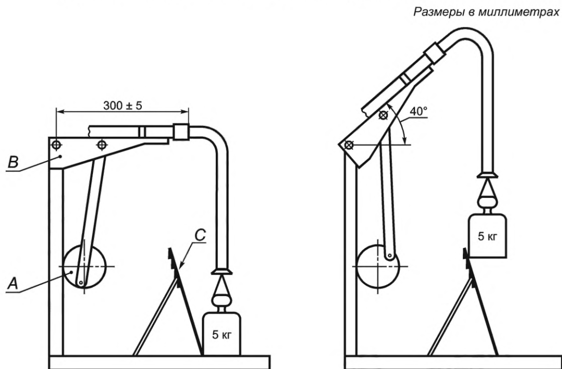
Рисунок 102 — Устройство для испытания токоведущих шлангов на истирание
