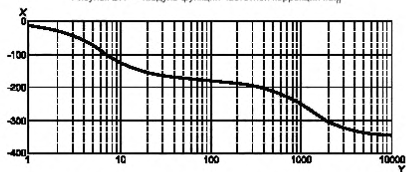
Рисунок D.1 — Модуль функции частотной коррекции flat_h
