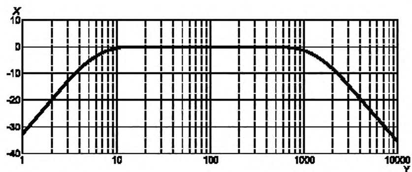
Рисунок D.1 — Модуль функции частотной коррекции flat_h
