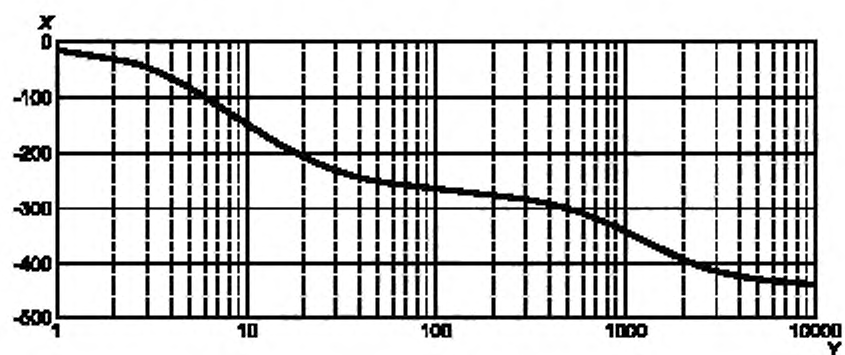
Рисунок E.1 — Модуль функции частотной коррекции W_h
