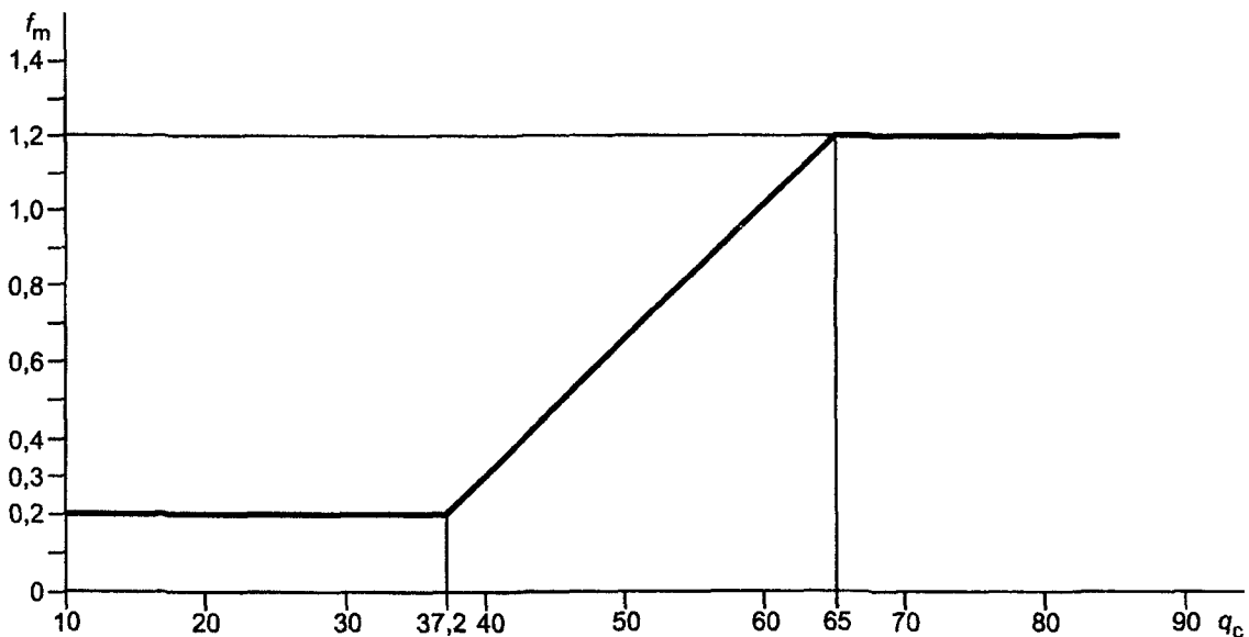
Рисунок 3 — Коэффициент дизеля f_m как функция приведенной удельной цикловой подачи топлива q_c
