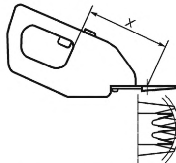
д) Рукоятка прикреплена спереди и сзади (соответствует 20.104)
