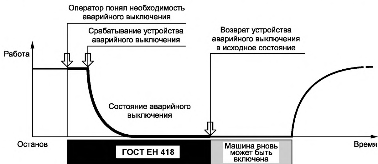
Рисунок 1 — Функциональные аспекты применения ГОСТ EN 418
